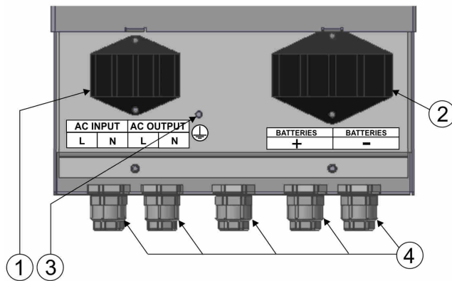
Widok czołowy
