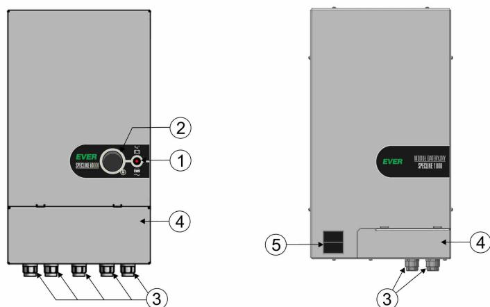
Zasilacz
