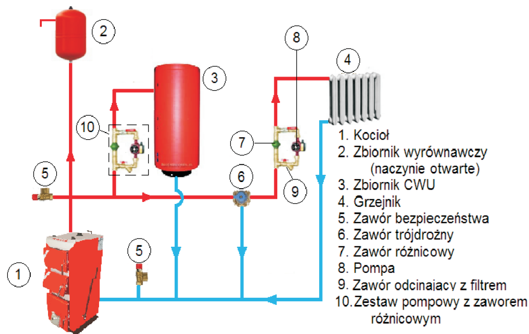
Rys. 2 Schemat podłączenia kotła
