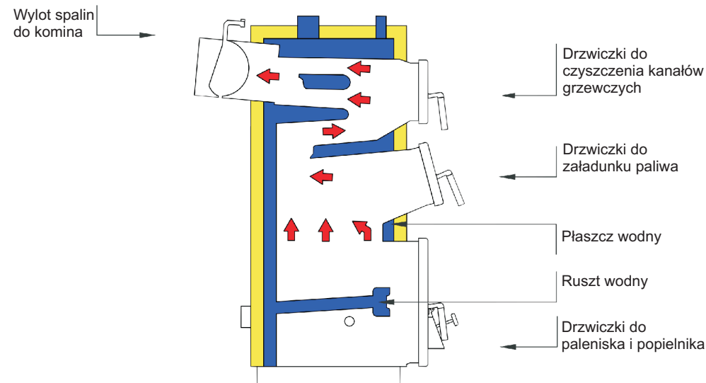
Rys. 1 Przekrój kotła
