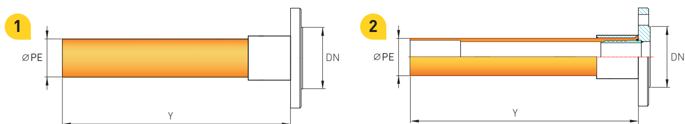
Połączenia PE/STAL z kotnierzem: SDR 17,6 RC
